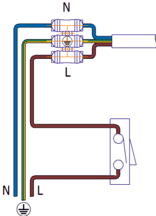
Kuva 1 - kytkentäkaavio
